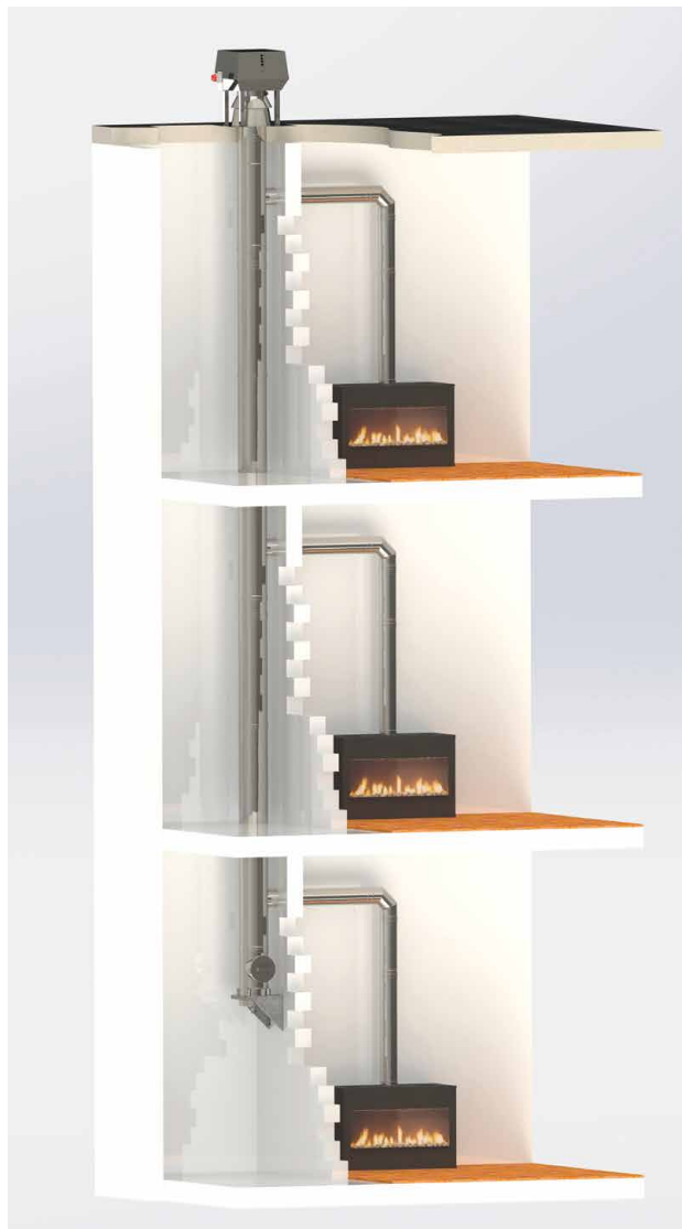
CSG-opstelling in onderdruk met concentrische aansluitingen 80/125 en collectieve ventilator op het dak.
