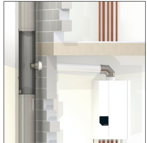
Aansluitelement naar de CV-ketel(s)
